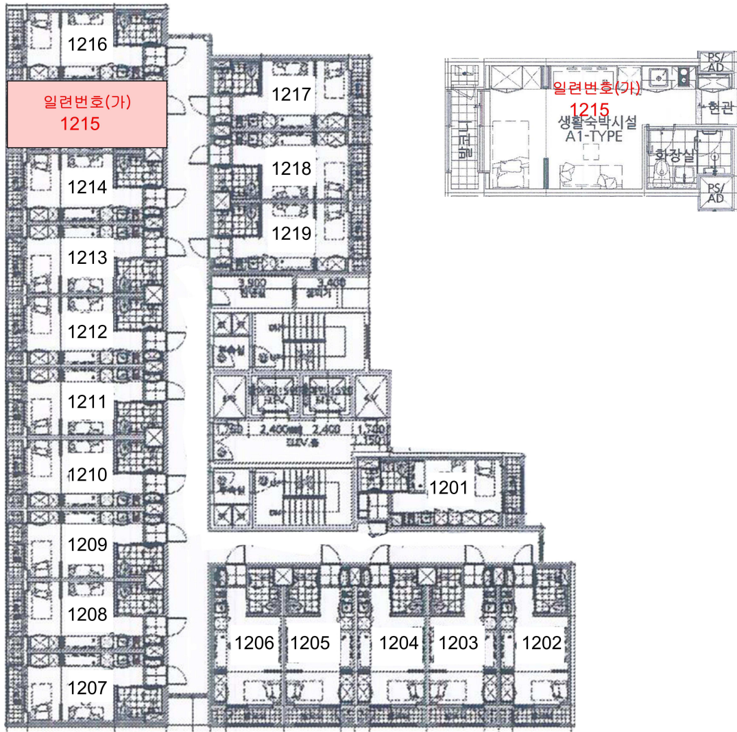
<내부구조도>
